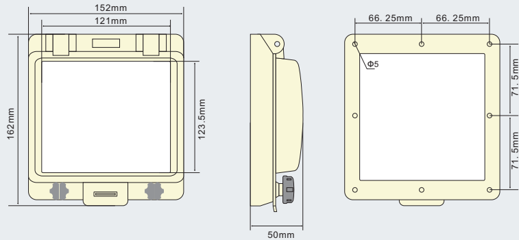
PWW-400K窗口产品外形尺寸、安装孔及孔位图
