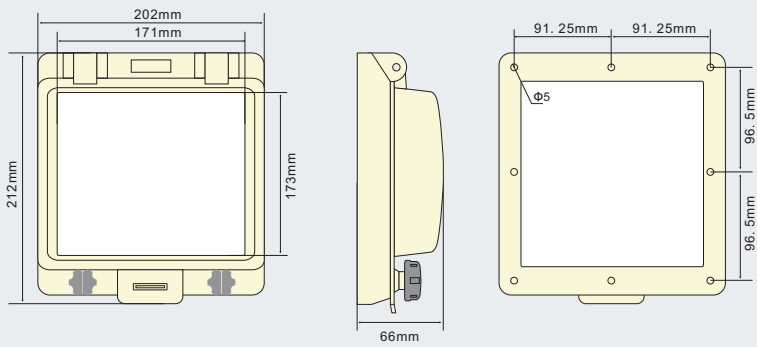
PWW-400K窗口产品外形尺寸、安装孔及孔位图
