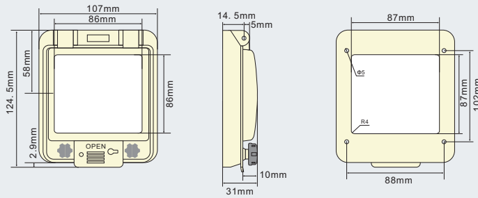
PWW-144K窗口产品外形尺寸、安装孔及孔位图
