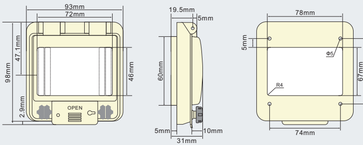
PWW-6窗口产品外形尺寸、安装孔及孔位图
