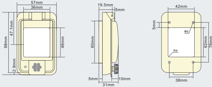
PWW-3窗口产品外形尺寸、安装孔及孔位图
