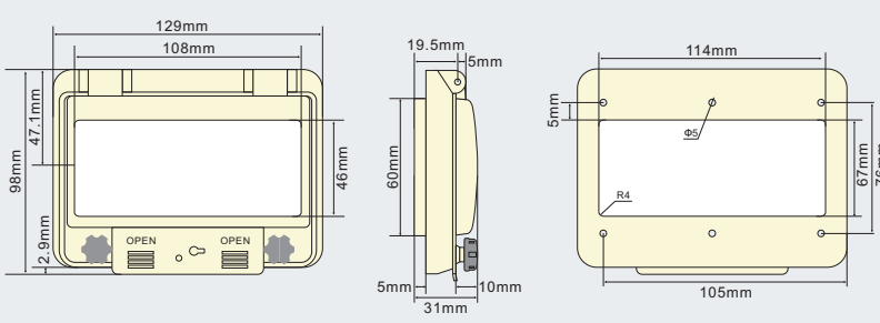
PWW-6窗口产品外形尺寸、安装孔及孔位图
