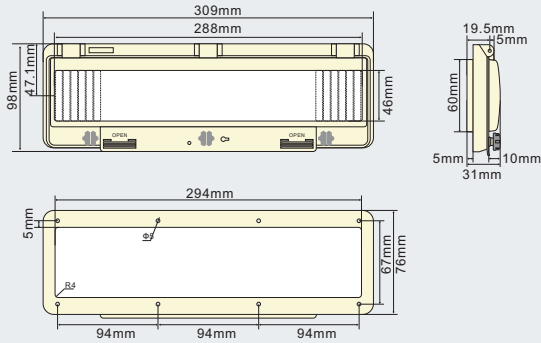
PWW-16窗口产品外形尺寸、安装孔及孔位图
