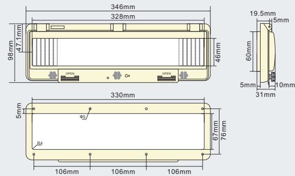
PWW-5窗口产品外形尺寸、安装孔及孔位图
