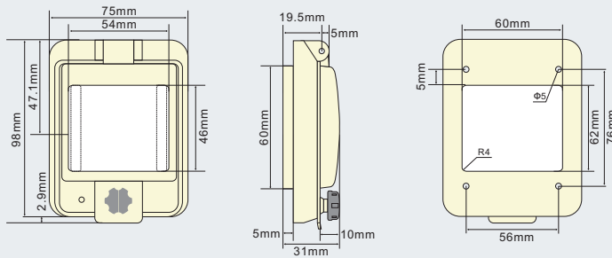
PWW-4窗口产品外形尺寸、安装孔及孔位图
