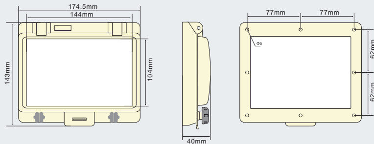
PWW-144K窗口产品外形尺寸、安装孔及孔位图
